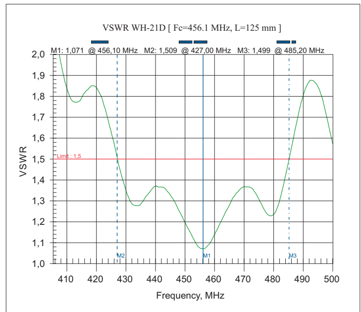
Typical VSWR test plots in VHF and UHF bands / Типовые графики измерений КСВн VHF/UHF
