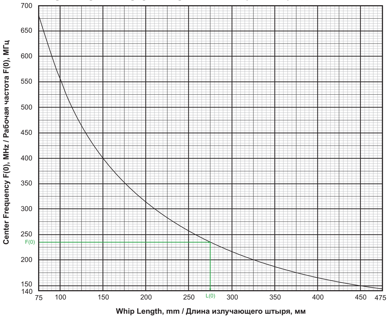
Whip Cutting Chart / График настройки на заданную частоту F(0)
